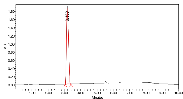
MS ESI(+) spectrum
