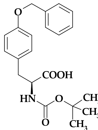
O-benzyl Boc-L-Tyrosine
