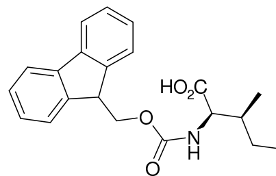
Fmoc-D- allo -Isoleucine
