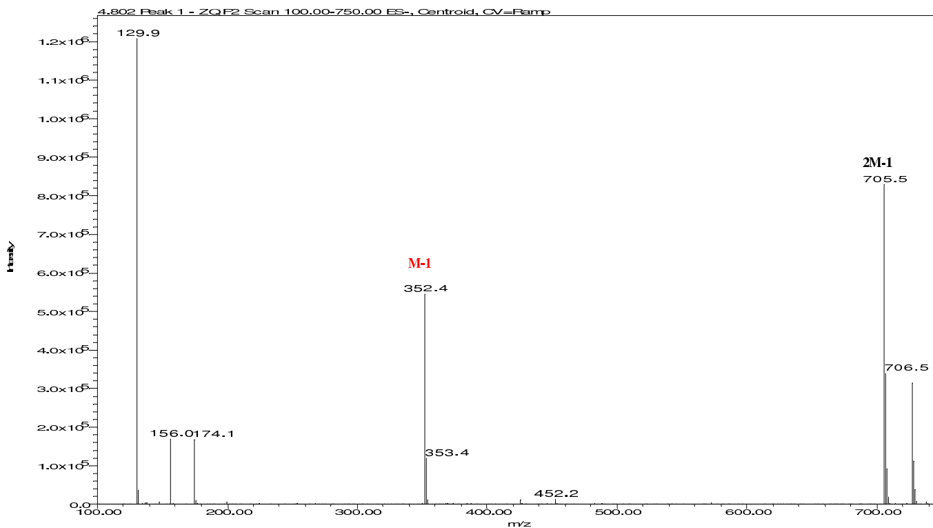
MS ESI(-) spectrum
