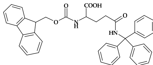
Fmoc-L-Glutamine(Trt)
