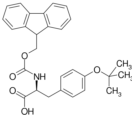
Fmoc-L-Tyrosine(tBu)
