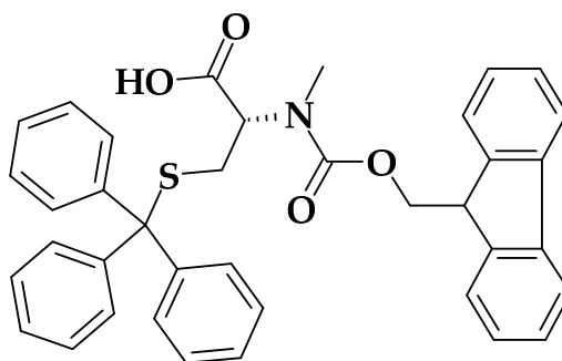
S-Trityl Fmoc-L-NMe-Cysteine
