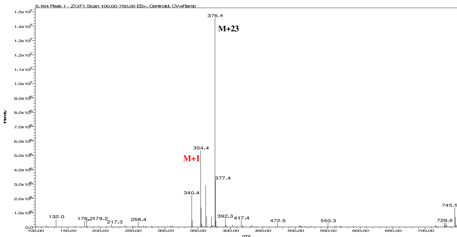
MS ESI(+) spectrum
