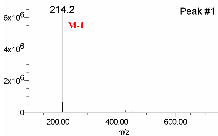
MS ESI(-) spectrum
