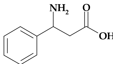
3-amino-3-phenylpropanoic acid
