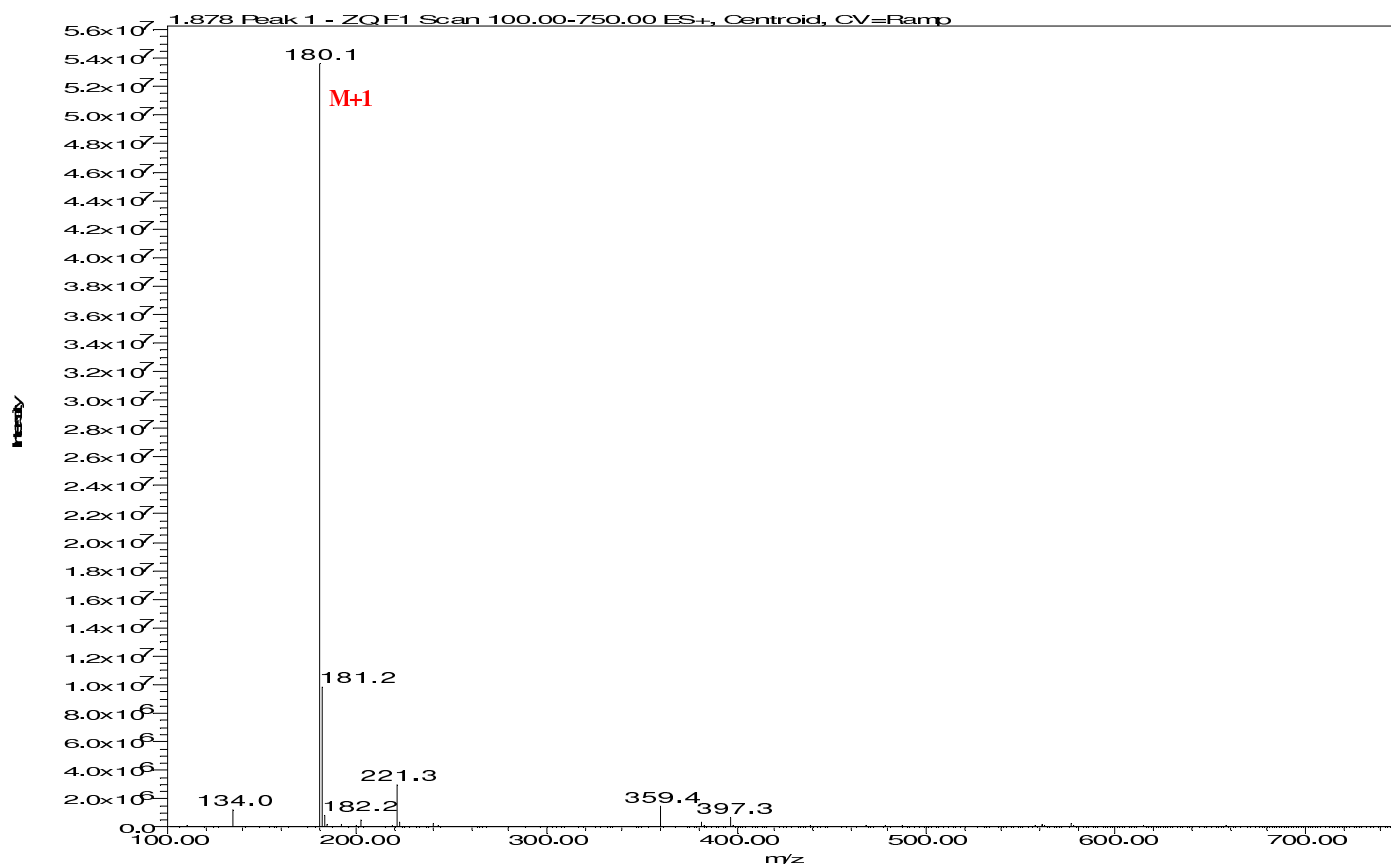
MS ESI(+) spectrum
