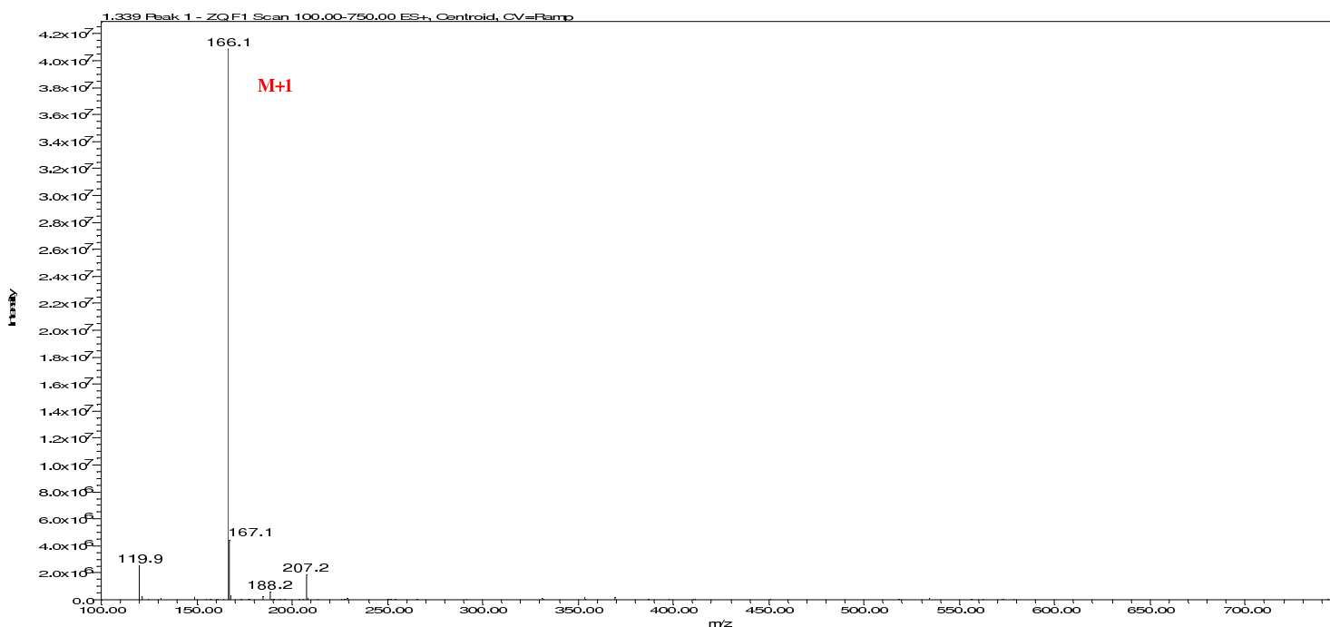
MS ESI(+) spectrum
