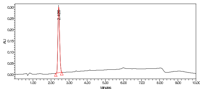
MS ESI(-) spectrum
