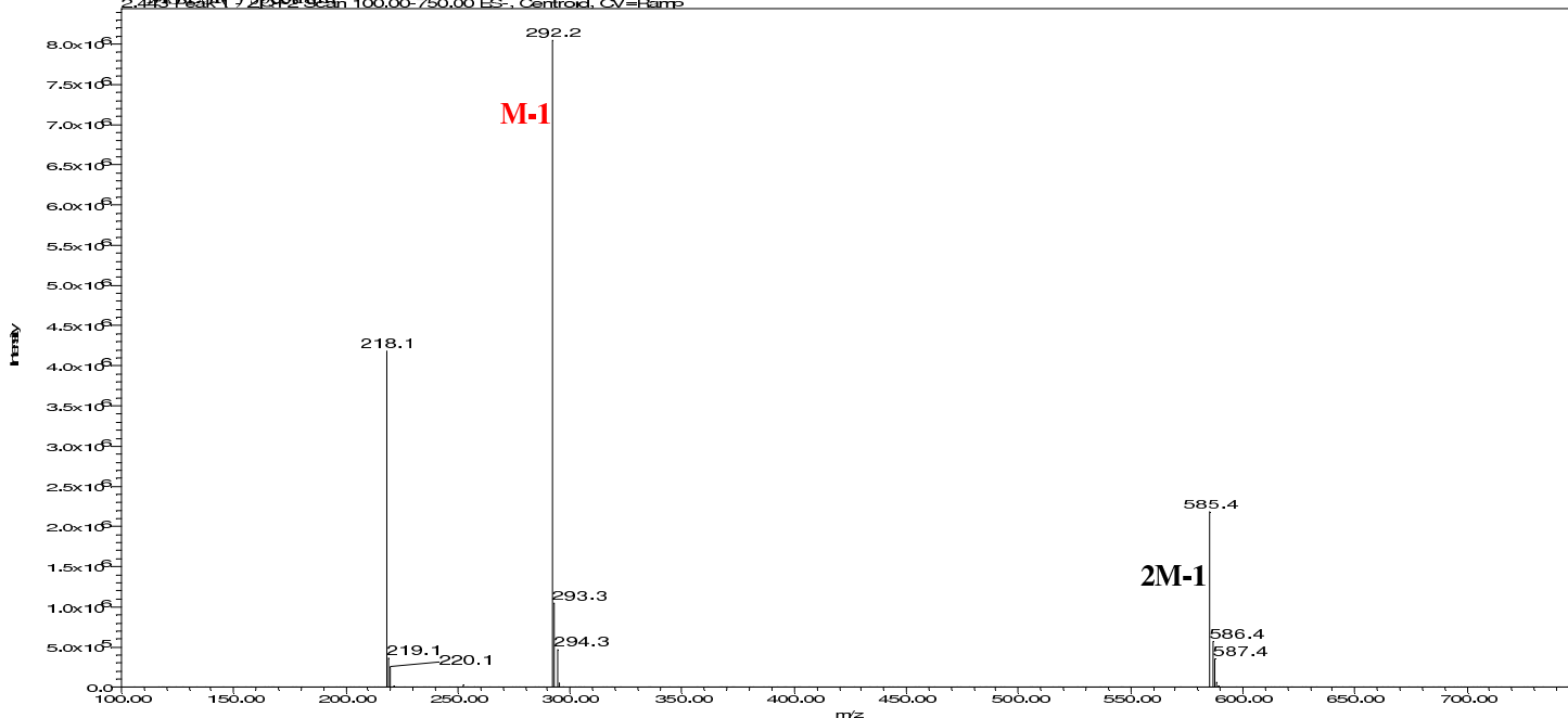
MS ESI(-) spectrum
