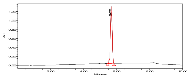
MS ESI(-) spectrum
