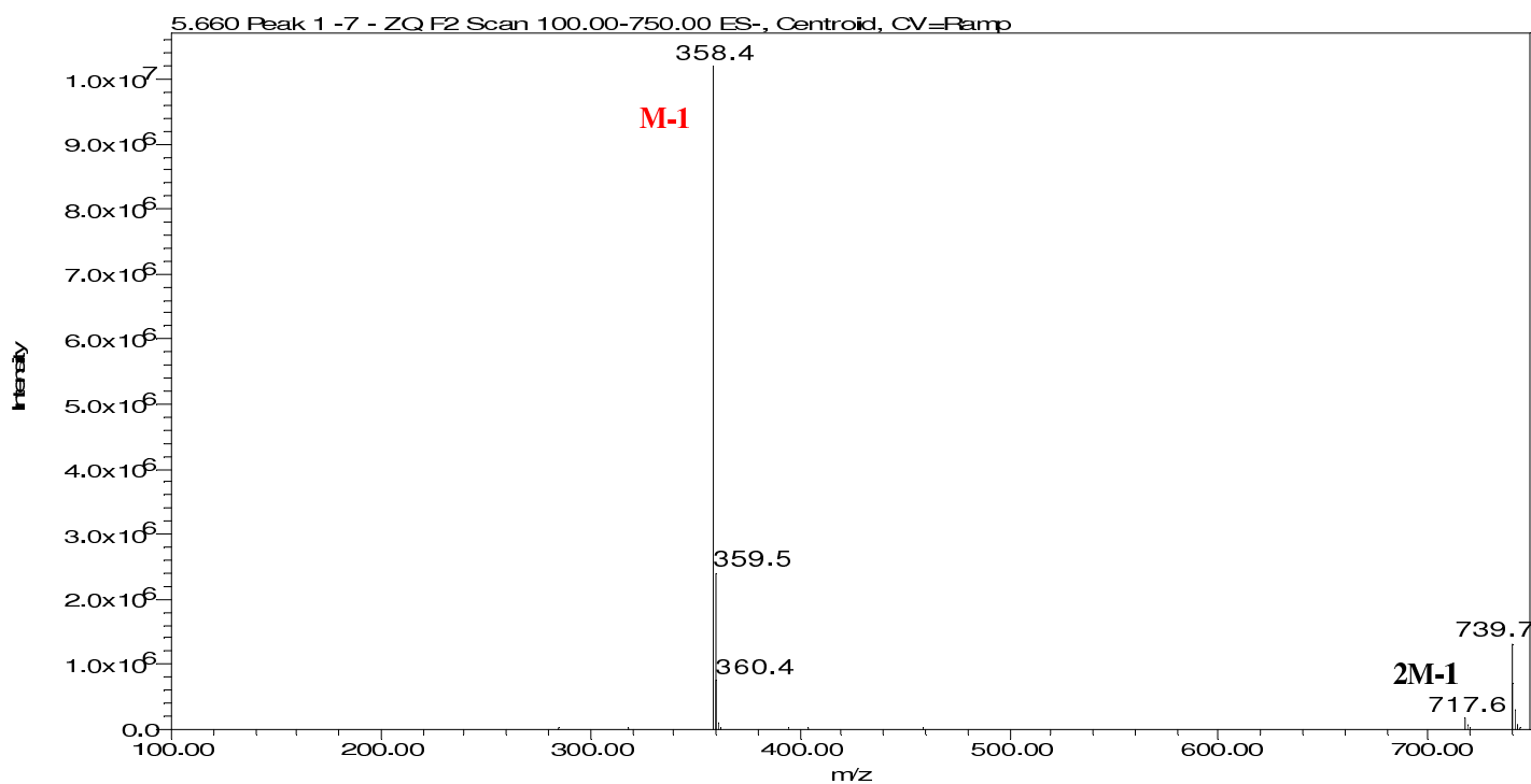
MS ESI(-) spectrum
