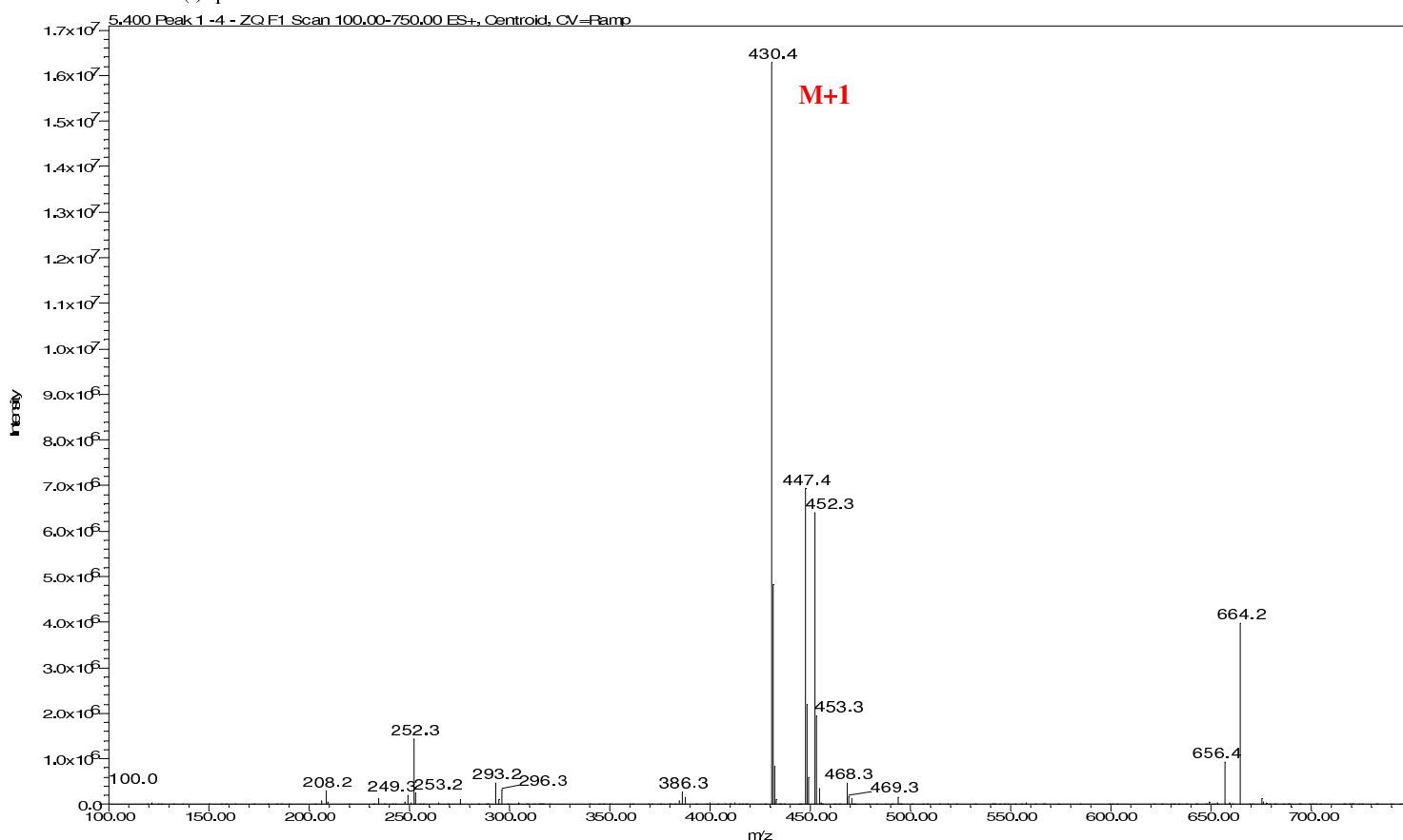
MS ESI(-) spectrum
