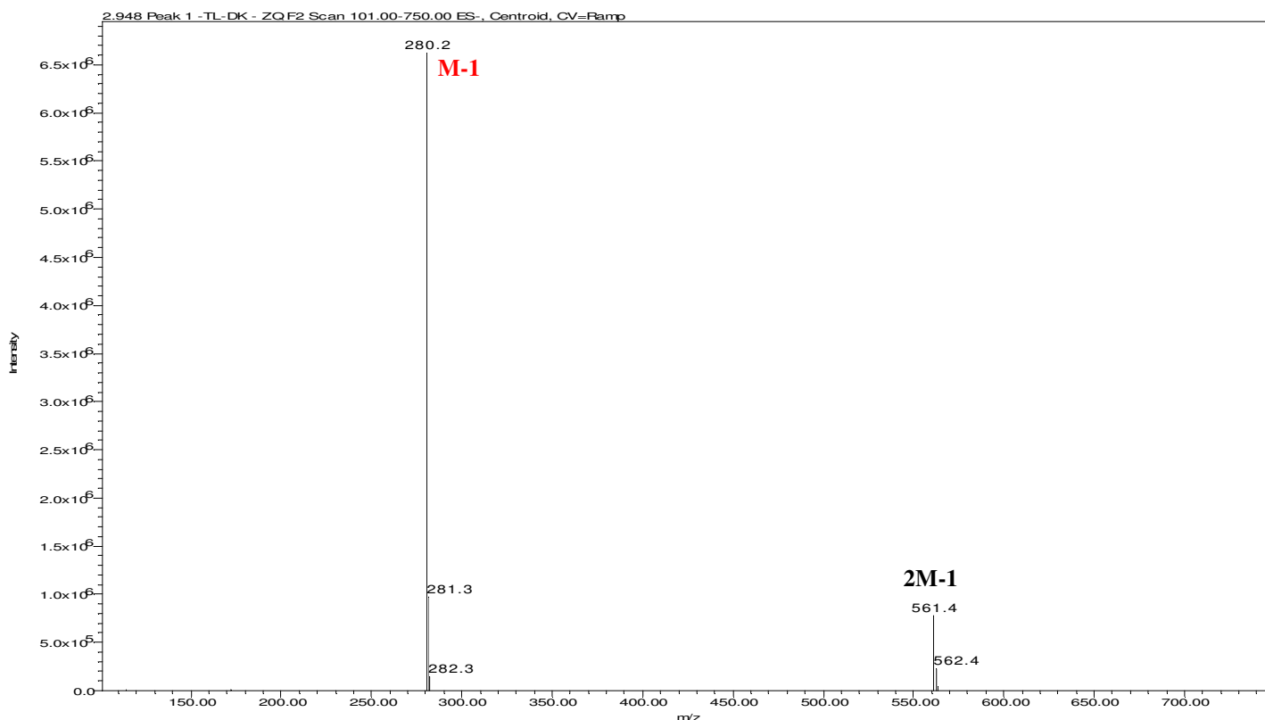
MS ESI(-) spectrum
