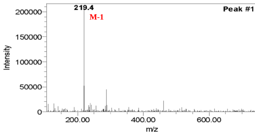
MS ESI(-) spectrum
